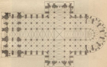
Grundriß des Kölner Domes.
