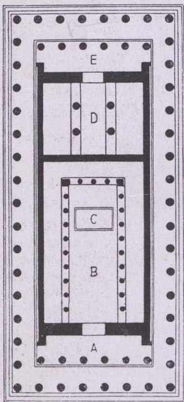
Fig. 38. Grundriß des Parthenon.
