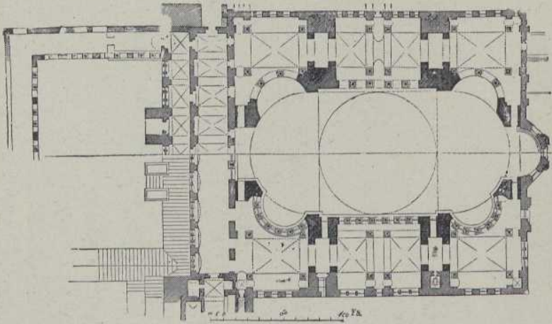
Abb. 6. Grundriß der Hagia Sofia in Konstantinopel.
