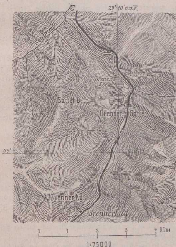
Fig. 12. Brennerbahn (Scheitel und Wasserscheide).
