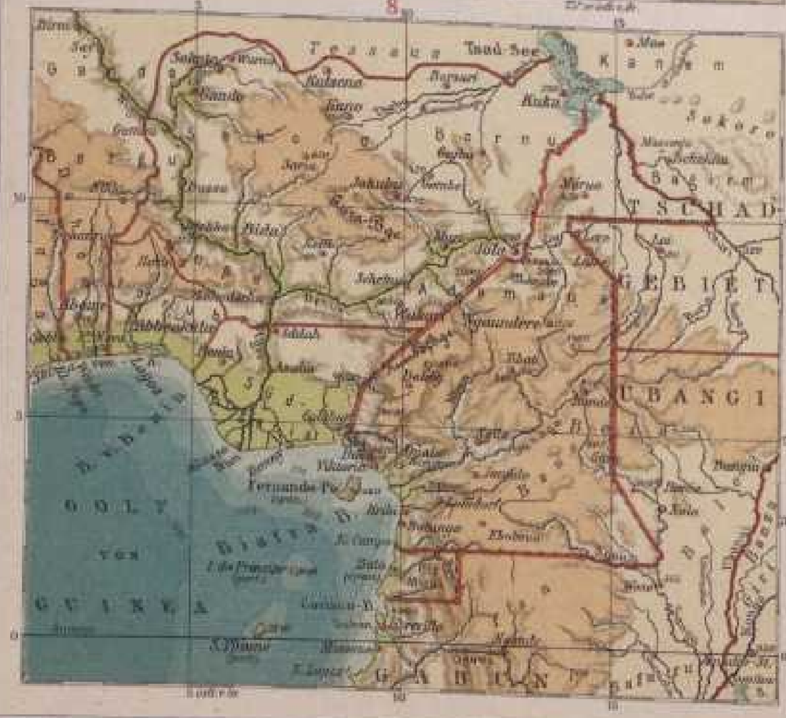
KAMERUN-GERIBGE OASE SUAH KANARISCHE INSELN (spanische Provinz) SANKT HELENA (brit.) KAPSTADT MIT DEM TAFELBERGE AMBRA-LANDSCHAFT (Abyssinien) UNTERLAUF DES KONGO LÄNDER AN DER RIAFRA-BAI DEUTSCH-OSTAFRIKA UND SANSIBAR Maßstab 1:1,500,000 Maßstab 1:1,500,000 Maßstab 1:5,000,000 Maßstab 1:750,000 Maßstab 1:750,000 Maßstab 1:750,000 Maßstab 1:10,000,000 Maßstab 1:20,000,000 Maßstab 1:20,000,000
