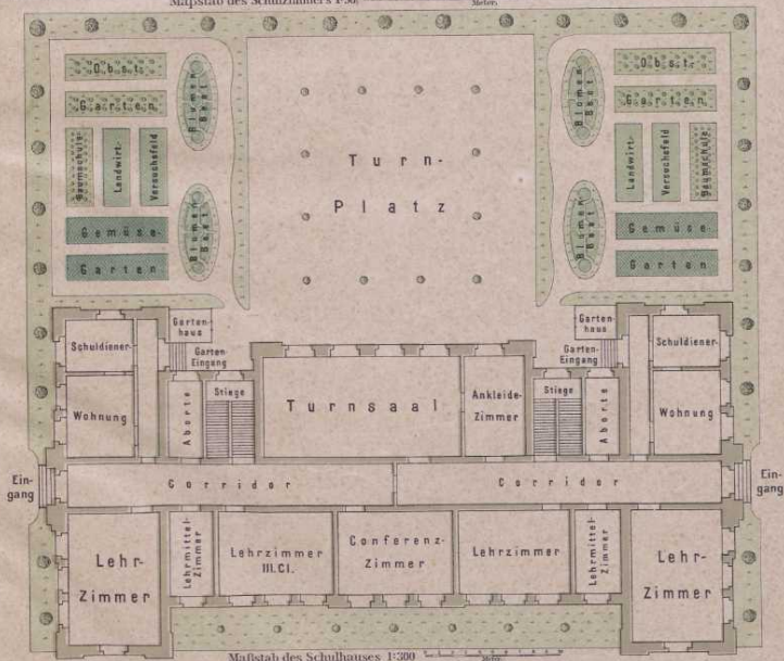
Maßstab des Schulhauses 1:300
