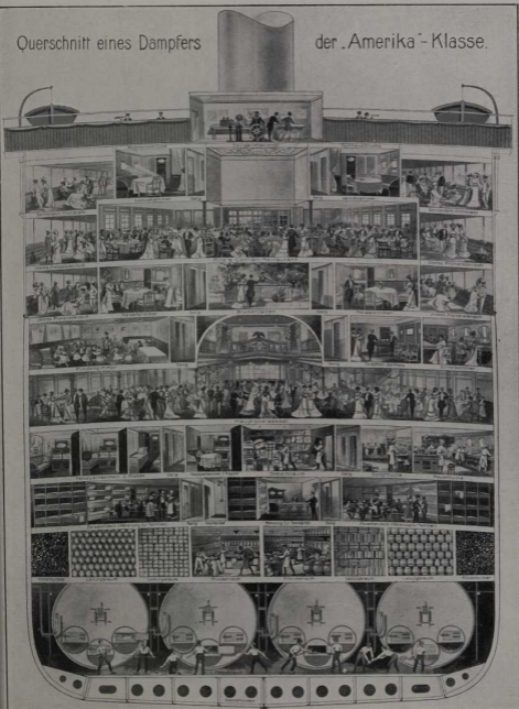
41. Querschnitt des Dampfers „Amerika“ der Hamburg-Amerika-Linie. Das Bild gewährt einen Einblick in den komplizierten Bau eines modernen Dampfers. Es zeigt, wie sich die hauptsächlichsten Passagiereinrichtungen, die Frachträume, die dem Schiffs- und Verpflegungsbetrieb dienenden Räume über die verschiedenen Decks verteilen und gibt so eine Vorstellung von der praktischen, zweckmäßigen Anordnung und der kunstvollen inneren Gliederung dieser Wunderwerke der Schiffbautechnik.
