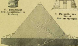
6. Pyramide des Cheops, Durchschnitt (mit der Grabkammer und dem Zugange).
