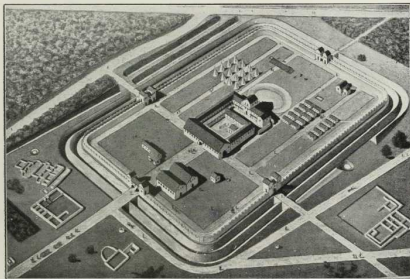
7. Die Saalburg bei Homburg v. d. S., aus der Vogelperspektive gesehen. (Wiederherstellung nach Jacobi, Das Römerkastell Saalburg .) Das Kastell ist 220 m lang und hat vier von Türmen flankierte Tore. In der Mitte befindet sich das Hauptgebäude, das Pædiorium, mit zwei Höfen, Exerzierhalle und Magazinen. Im engsten Schutzbereich des Kastells, unmittelbar vor den Mauern, hatte sich eine Lagerstadt aus Marktenderwohnungen und Wirtschaftshäusern gebildet. Auch Reste eines Heiligtums des Mithras und eines Friedhofes wurden bei den Ausgrabungen entbedt.
