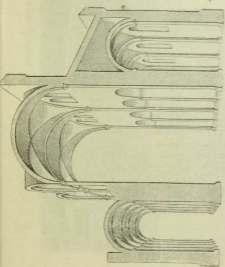
Fig. 88. Romanisches Kreuzschiffen. § 57, 1.
