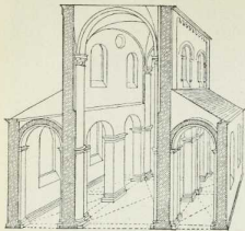
Romanisches Gewölbesystem. (H. Watzki, Bauk., Taf. 1.)
