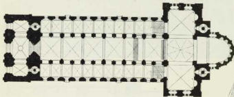
Dom zu Speyer (Grundriß). (H. Zehn und v. Seyd.)
