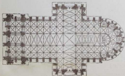
Fig. 177. Der Grundriß des Cölnner Doms.
