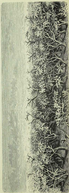
Fig. 14. Scrubgebiet oder Busch in West-Australien. (Die Zahl der abgetrockneten Bäume übersteigt oft diejenige der lebenden.) — S. S. 61.
