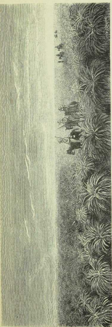
Fig. 13. Stachelschwanzgras (Scaevola)-Wüste Inner-Australiens. — S. S. 61.
