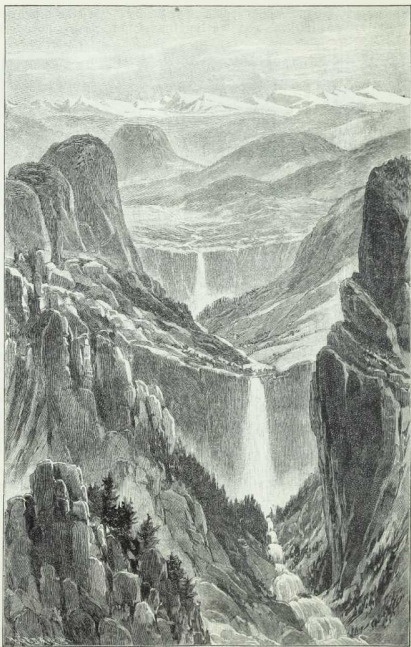
Fig. 38. Das Yosemite-Tal. Das Tal ist gegen 25k m lang, seine Felswände sind 1000 bis 1300 m hoch. An seinen Eingängen stehen Granitfelsen von merkwürdiger Gestalt bis 1100 m hoch. In ihm Wasserfälle von 600 bis 850 m Höhe. Die Talsohle liegt 1800 m über dem Meere.
