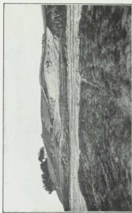
8. Düne im Bartischbruch bei Adelnau. (Phot. Prof. Dr. Pfabl, Polen.)
