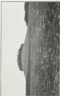
5. Bismarckkopf bei Erün. Endmoränenkuppe. (Phot. Direktor Dr. Schjerning, Berlin.)
