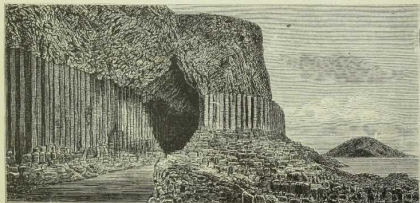
Säulenförmige Bildungen aus Basalt: Fingalshöhle auf der Insel Staffa.
