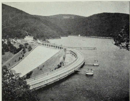
No. 48. Die Urfttalsperre bei Gemünd in der Eifel. (Photograph. Verlag Wilh Lenz in Gemünd.)
