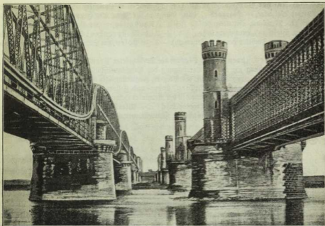
Abb. 2, § 70. Weichselbrücken bei Dirschau, 837 m lang, also doppelt so lang wie die Hamburger Elbbrücke. (Verlag W. Kraus, Dirschau.)
