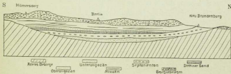
Profil durch das Norddeutsche Tiefland bei Berlin. (Nach Walther.)
