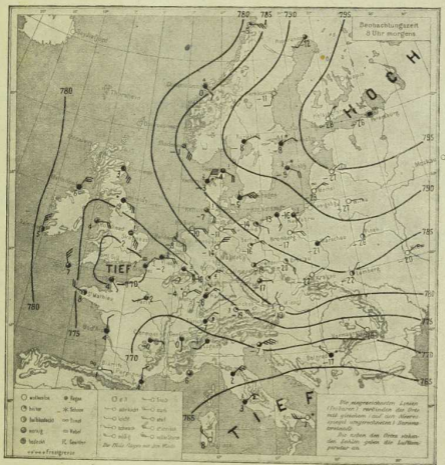
Wetterlage in einem Hochdruckgebiet.
