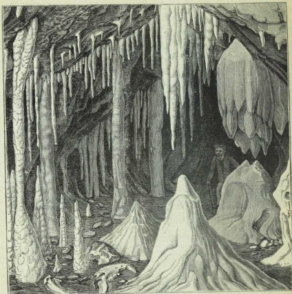
Fig. 17. Tropfsteinhöhle aus dem älteren Kalkgebirge. Aus der Hermannshöhle bei Rübeland im Harz. S. S. 10 und 37. Im Vordergrund Unterkiefer und Schenkelknochen des Höhlenbären.
