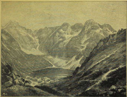
Die Hohe Tatra in den Karpathen. (Hölzel, Geogr. Charakterbilder, Fischsee und Meeraugespitze.)
