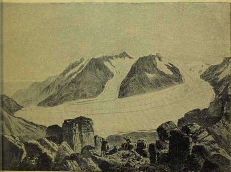
Der Aletschgletscher, der grösste Alpengletscher. (Lehmann, Geogr. Charakterbilder.)
