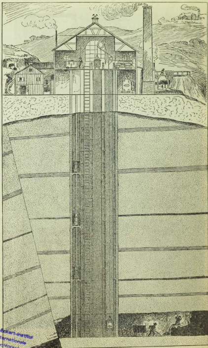
19. Durchschnitt eines Bergwerkes.
