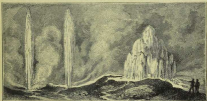
9. Heiße Quellen: Geysir auf Island.
