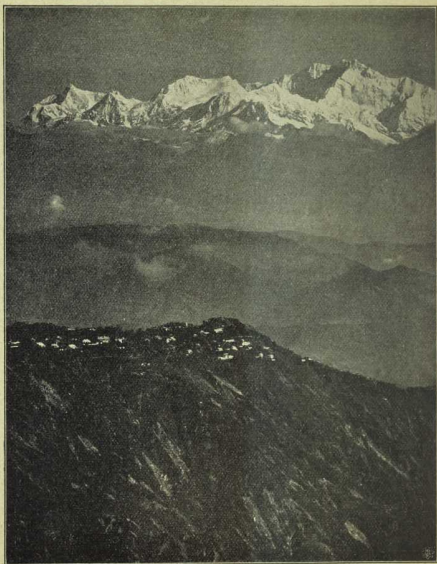
Abb. 1, § 37. Blick auf das Himalajagebirge von Darbshiling aus. (Aus Grube, Geographische Charakterbilder , Bd. 2. 29. Aufl.)
