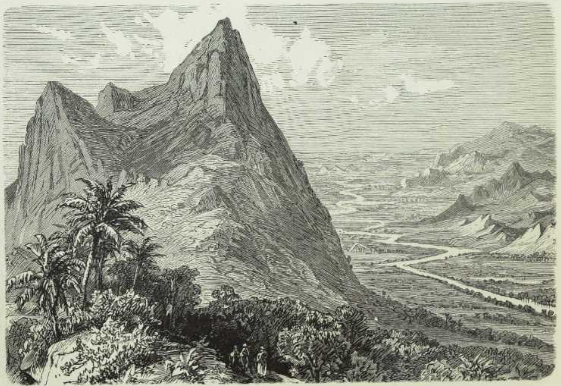
Der Myit-Ugeh, östlicher Quellfluß des Irawadi. (Nach V. Langlois.)
