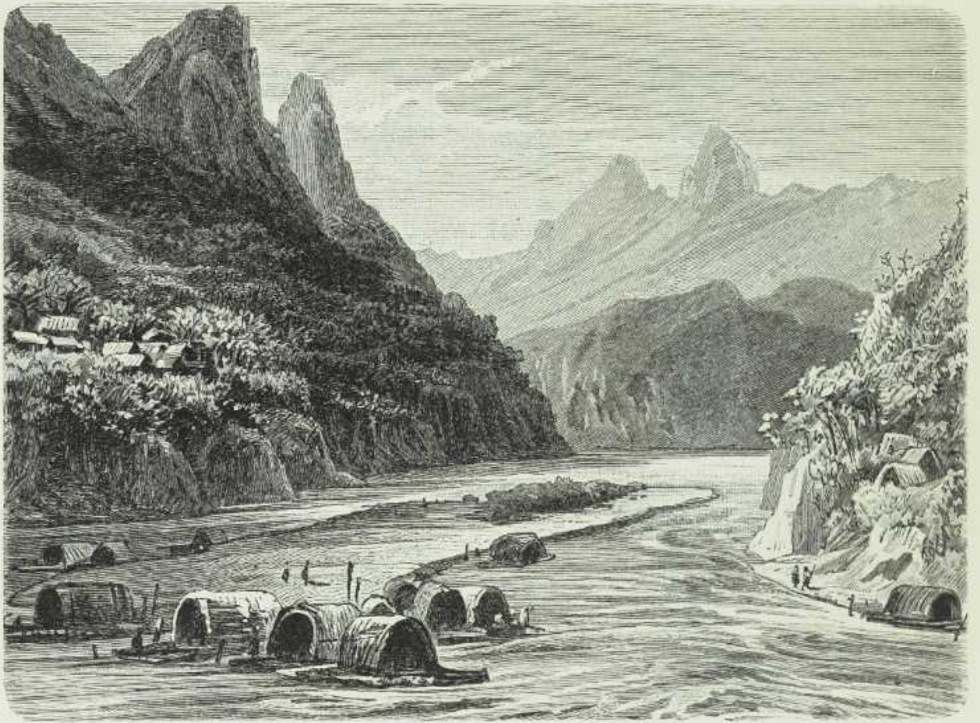
Thal des Nam-U am oberen Mekong. (Nach P. Reiss.)
