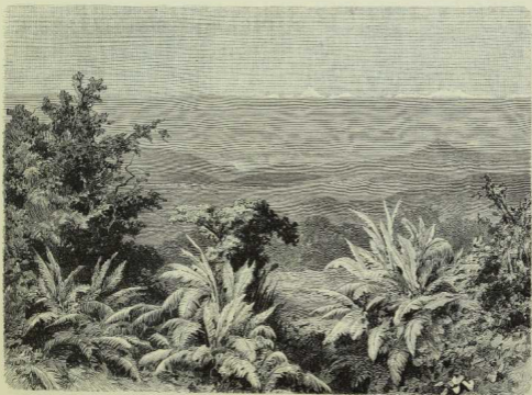
Thalweg des Magdalenaflusses bei Umbalema in Columbia. (Nach M. v. Thielmann.)
