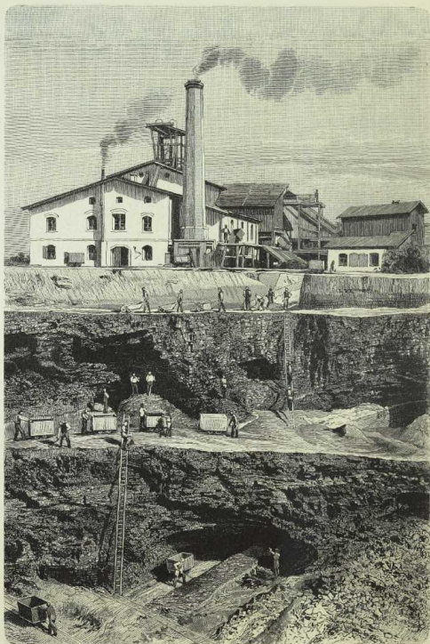
Braunkohlentagbau bei Dux in Böhmen. (Nach Photographie.)
