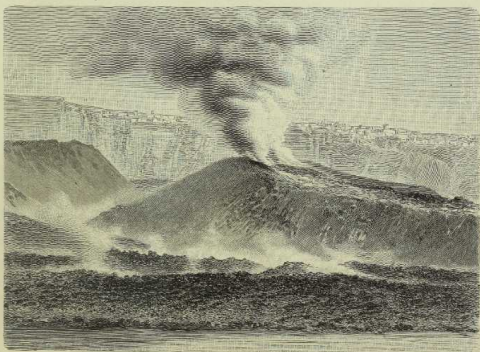
Der Thera-Krater auf Santorin. (Nach Photographie.)
