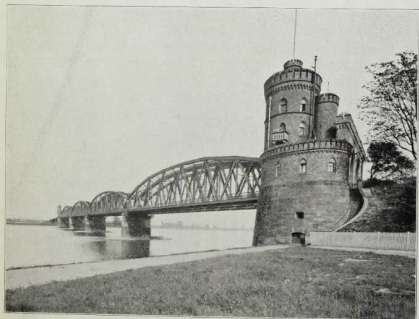
Rheinbrücke zwischen Gustavsburg und Mainz. (Ansicht nach dem Umbau in den Jahren 1911 und 1912). Seite 10.
