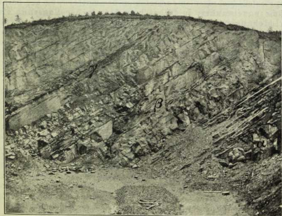
Fig. 68. Steinbruch im Mitteldevon mit drei verschiedenen Ablagerungen.
