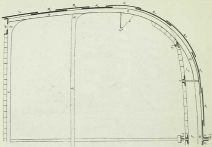
Fig. 7. Halber Querschnitt eines eisernen Schiffes. Auch Wülsteln, Zemannschiff. — Querschnitte befinden sich auf dem Klappbrett am Ende des Bilderrahmens.
