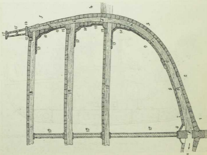
Fig. 8. Halber Querschnitt eines hölzernen Schiffes. Auch Wülsteln, Zemannschiff. — Querschnitte befinden sich auf dem Klappbrett am Ende des Bilderrahmens.
