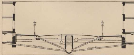
h. Querschnitt des Straßenunterbaues in einer modernen Stadt.
