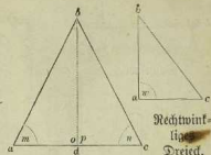
Gleichseitiges Dreieck.
