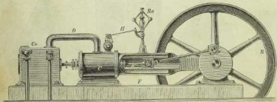
Dampfmaschine.
