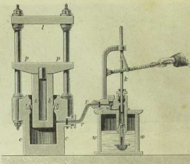
Hydraulische Presse.
