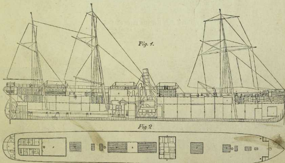
Längenschnitt u. Deckriß des Baarendampfers „Pollux“ (Eigenthum des österreichisch-ungarischen Lloyd.)
