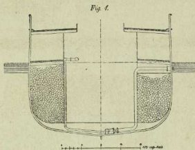
Querschnitt des „Pollux“.
