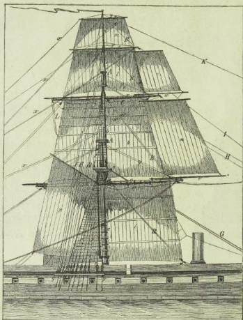
Großmast einer Corvette unter allen Segeln.
