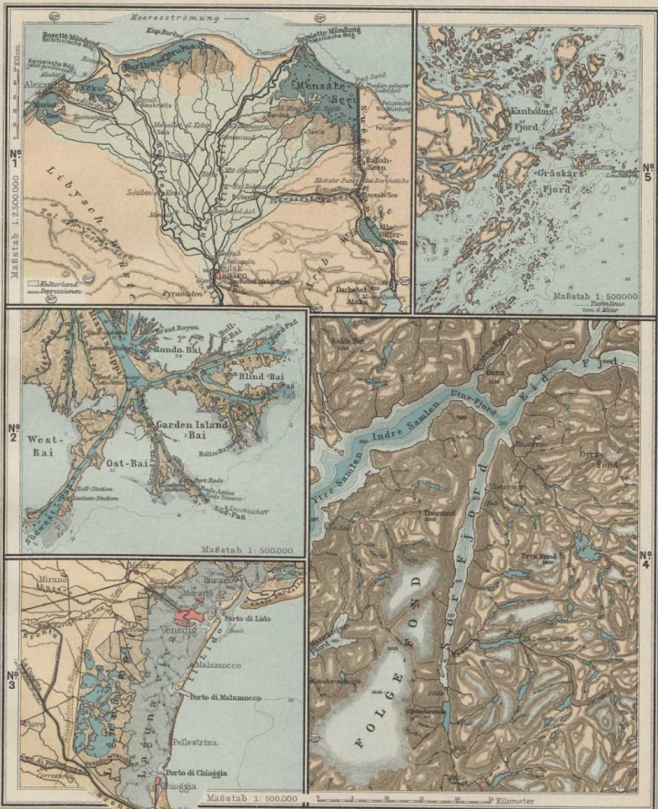
Nº1 Ausfüllungsdelta (NU) Nº2 Vorgeschoenes Delta (Mississippi) Nº3 Flachküste mit Lagune (Lagune von Venedig) Nº4 Steilküste und Fjordlandschaft (Hinterer Hardanger Fjord) Nº5 Schärenlandschaft bei Stockholm
