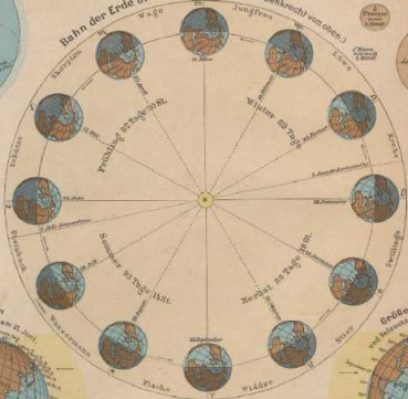
Tageslängen
