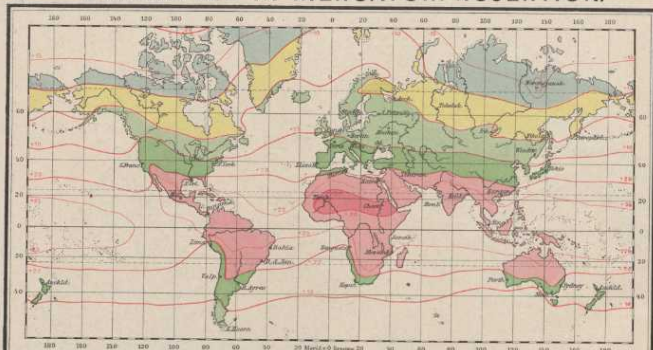
Jahres-Isothermen.
