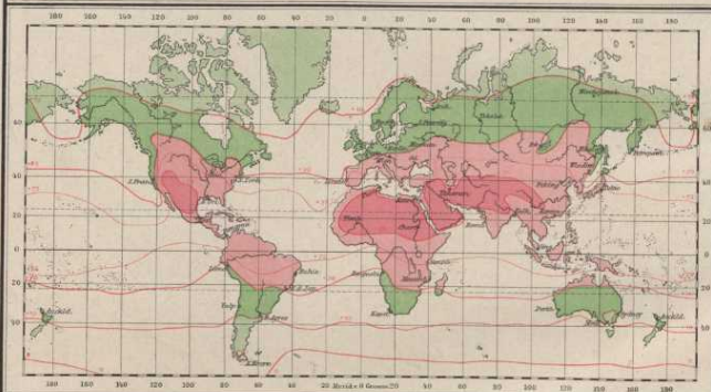
Juli-Isothermen.
