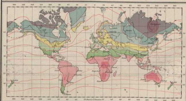
Januar-Isothermen
