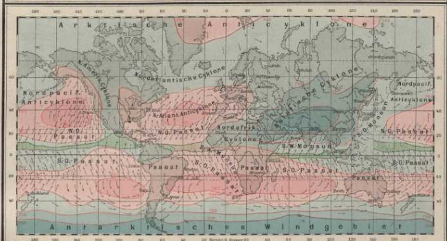
Luftdruck und Winde im Juli.
