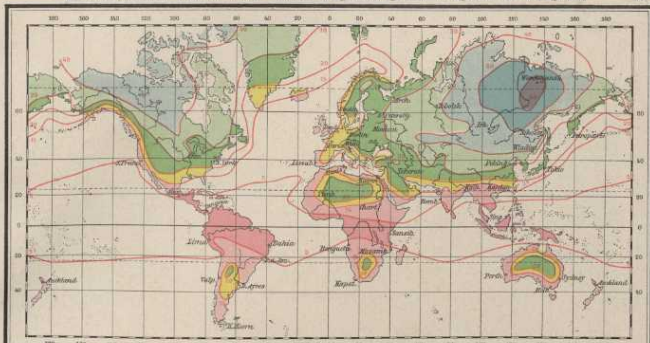
Linien gleicher Wärmeschwankung.
