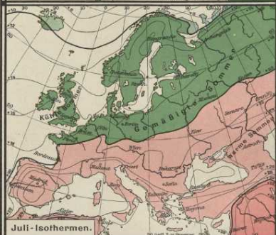
Juli-Isothermen.
