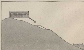
Aufriß der Walhalla.
