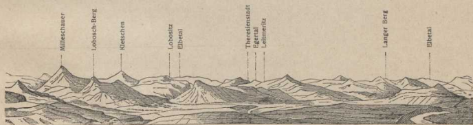
Das böhmische Mittelgebirge (nach Hochstetter). (Atlas S. 6/7.) (Beispiel eines Kuppen- oder Kegelgebirges.)
