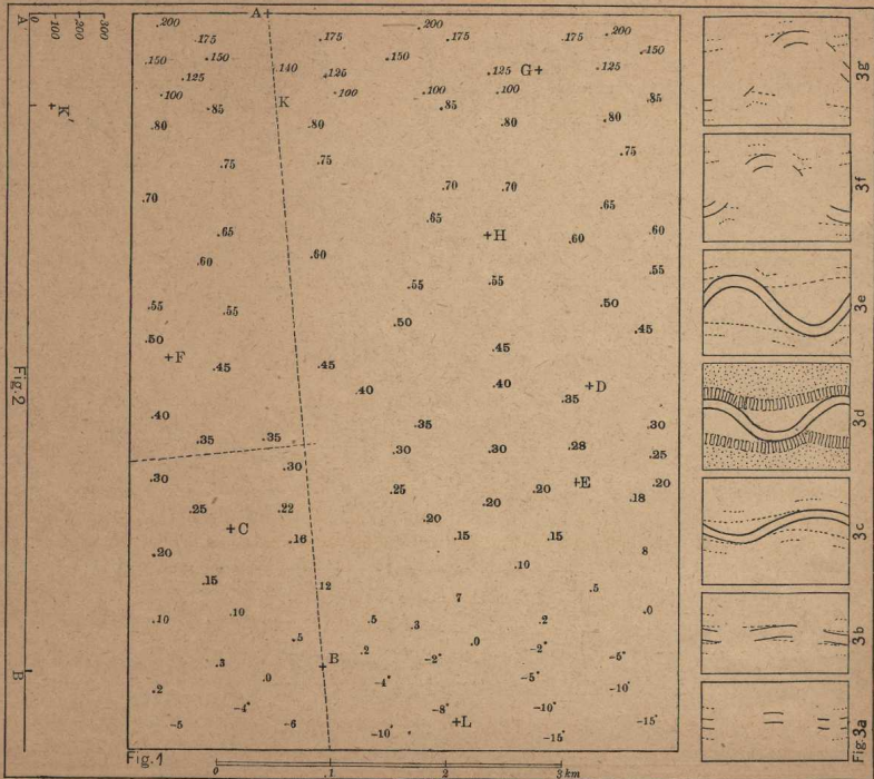
Fig. 1 und 2. Höhenziffernkarte und Profil einer Küstenebene.
