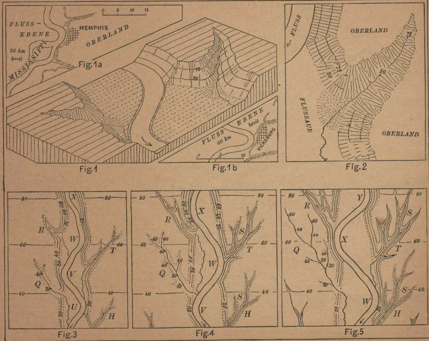
Fig. 1—5. Die Entwicklung der Täler in einer Küstenebene.
