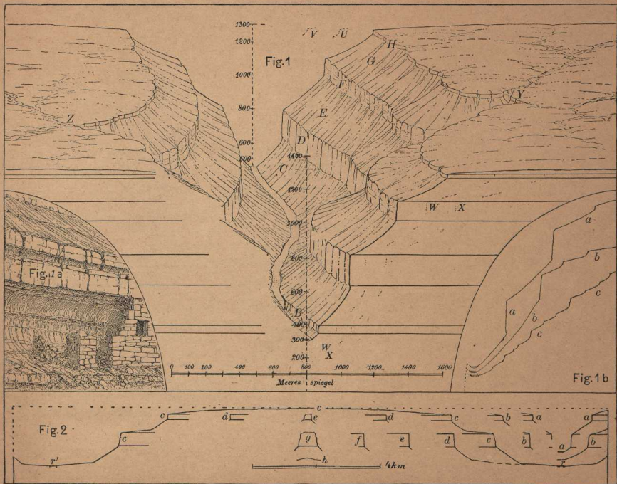
Fig. 1. Cañon im Tafelland (weiteres Entwicklungsstadium).
