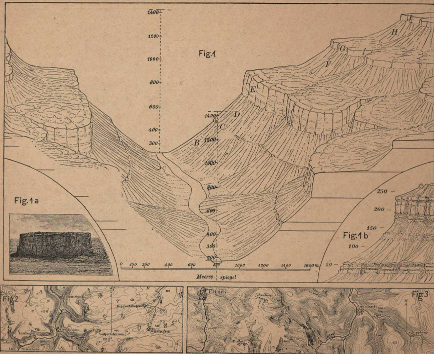
Fig. 1 a und b. Details von der Oberfläche und dem Abfall eines Tafellandes.
