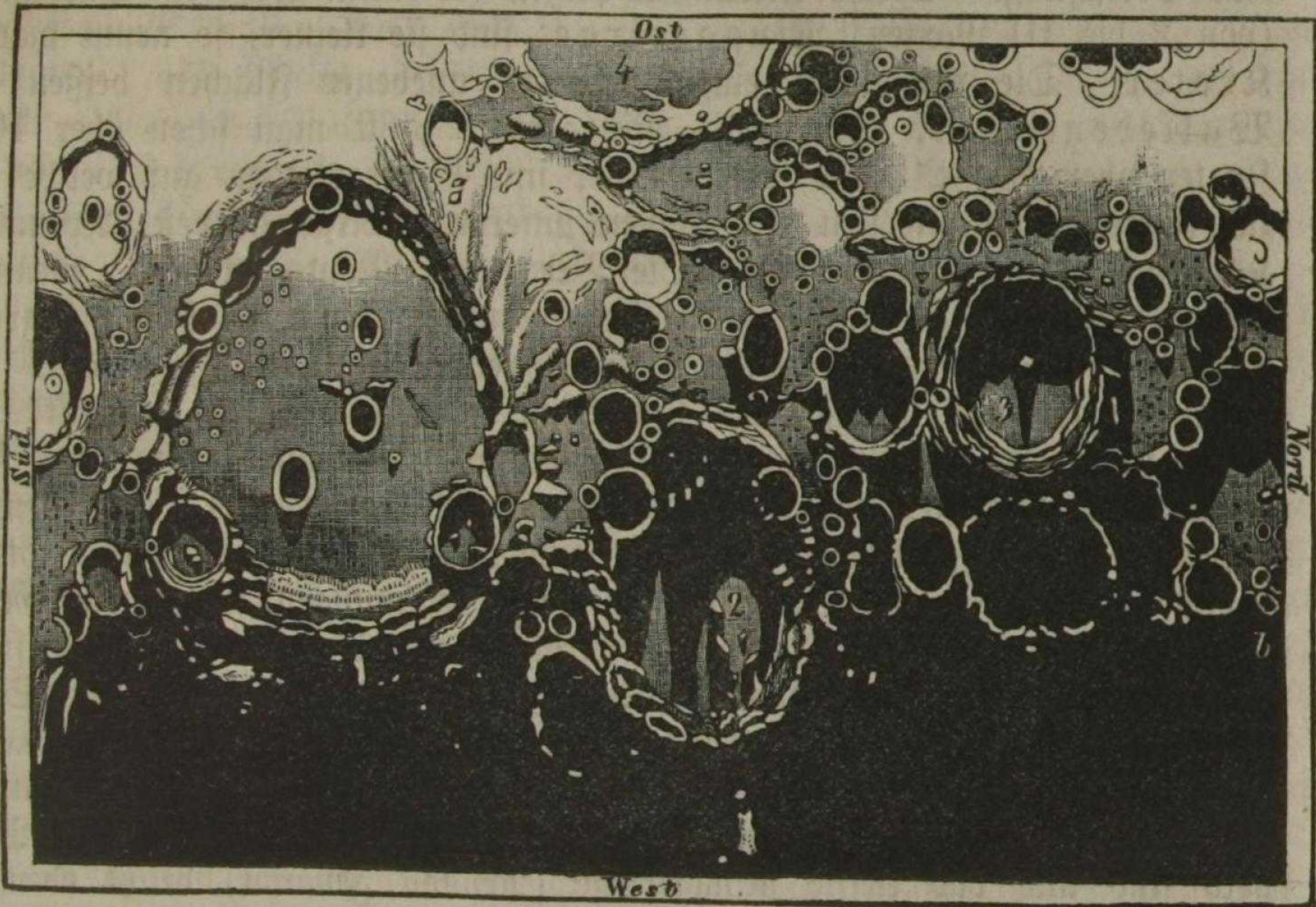
Schattenwurf der Kraterlandschaft des Mondes um Tycho bei untergehender Sonne. 1 die Wallebene Clavius; 2 die Wallebene Maginus; 3 der Krater Tycho; 4 die Wallebene Longomontanus; ab die Richtung der Lichtgrenze.
