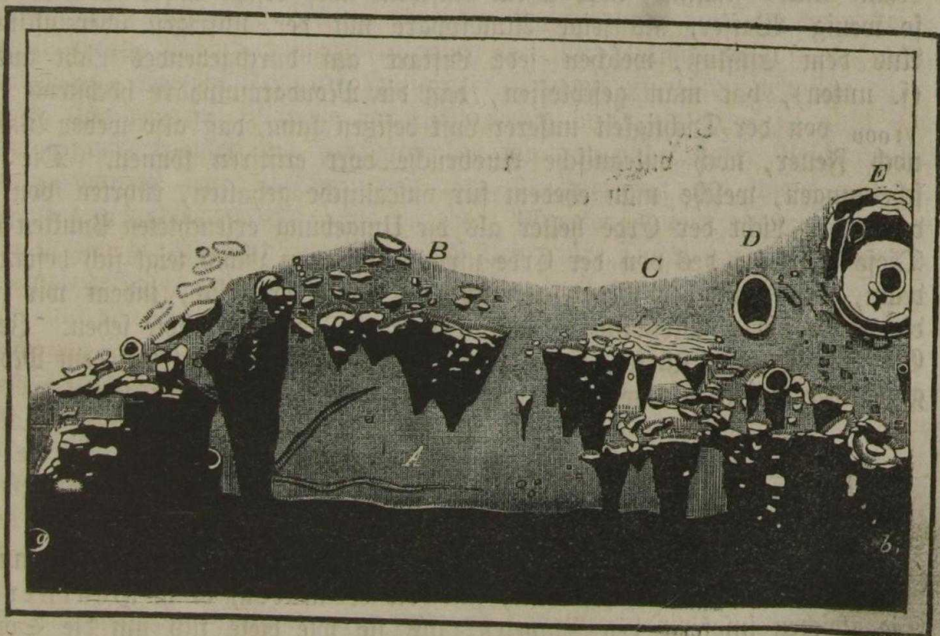
Schattenwurf des Mondgebirges Kaukasus bei untergehender Sonne. A das mare serenitatis; B der südliche Theil des Kaukasus; C der nördliche Theil; D Krater Thenetetus; E das Ringgebirge Cassini; ab die Richtung der Lichtgrenze.
