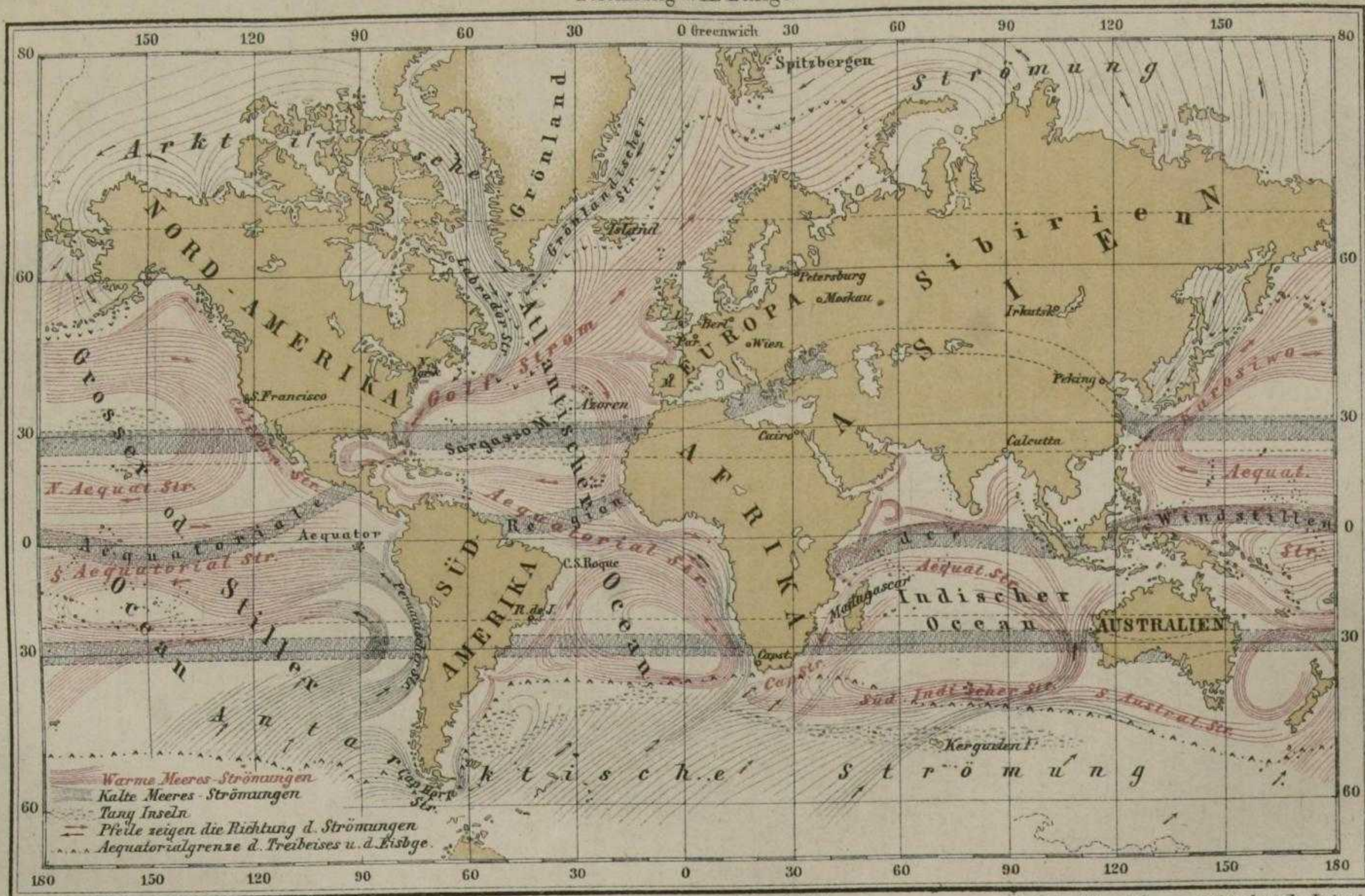
Fig. 39. MEERESSTRÖMUNGEN. Zeichnung v. H. Lange.
